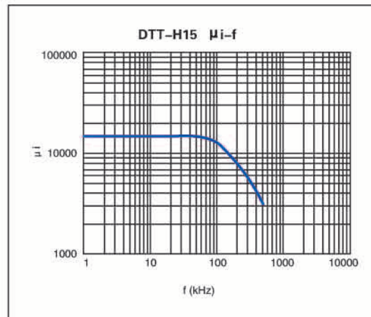
\mu -f 特性曲线 \mu -f characteristic curve
